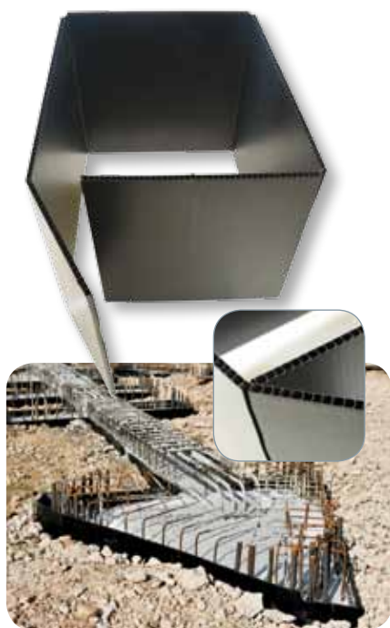
Semelles, massifs et réservations
