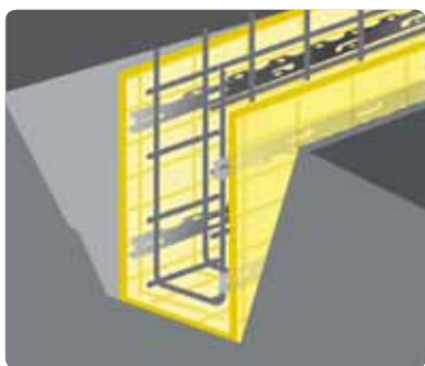
❶ Placement des armatures et des distanciers en plastic profil type A
