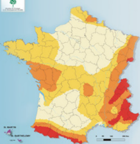
Aléa sismique de la France
